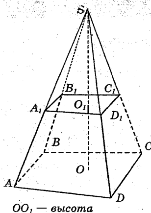
OO_1 — высота
