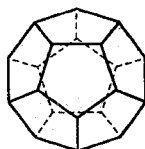
Додекаэдр
