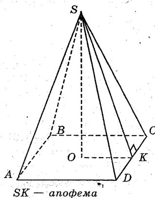
SK — апофема
