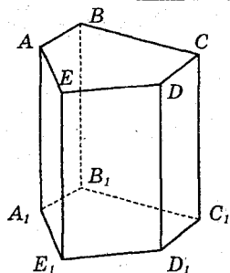
Прямая призма
